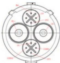
IEC62196-3: CHAdeMO
